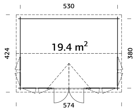
Doppelverglast
