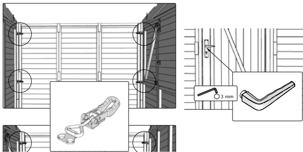
Spannverschlüsse arretieren und den Türgriff montieren
