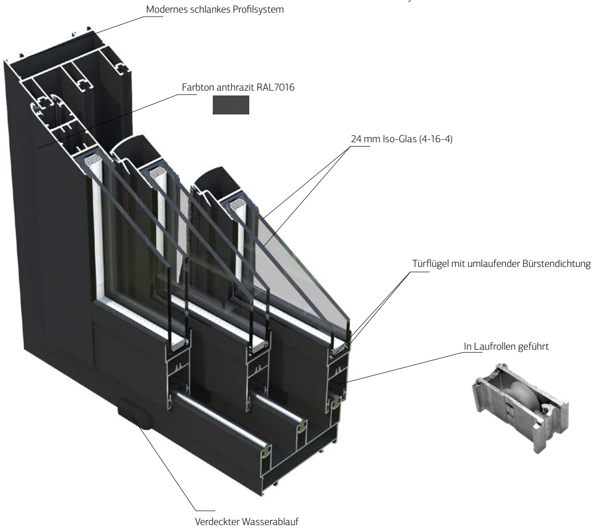
Alu-Schiebetürsystem mit zwei oder drei Glaselementen
