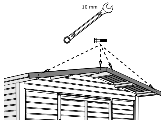
Blendbretter montieren
