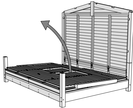
Wandelemente aufrichten
